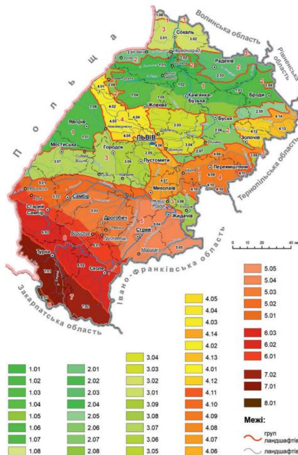
Рис. 2.8. Ландшафтна карта Львівської області
