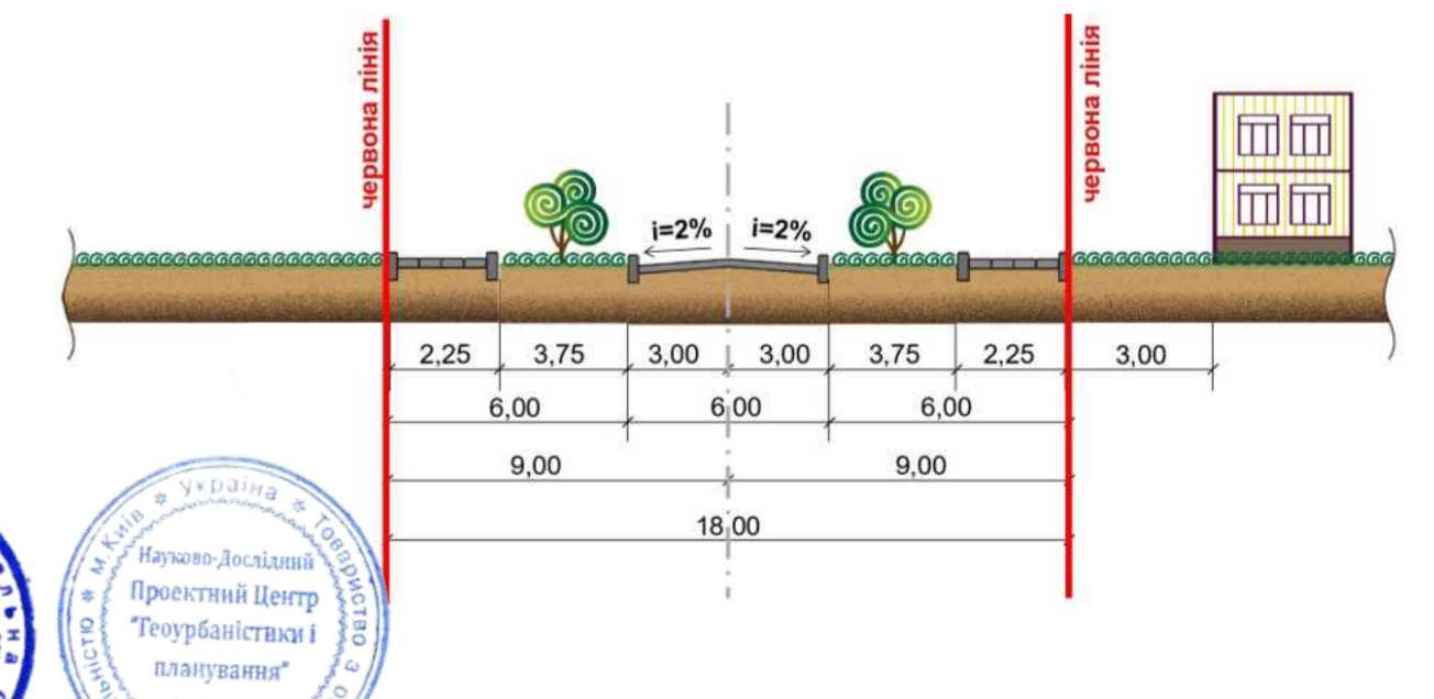
Профіль 1-1 вул. Героїв УПА та вул. Івана Франка
